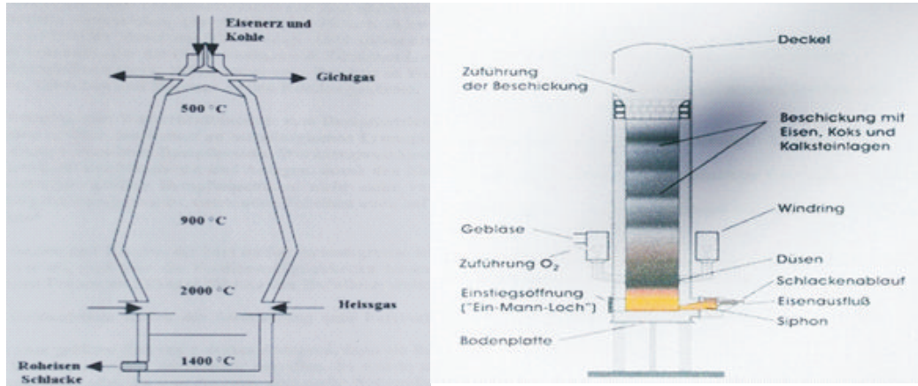
Schematische Darstellung der zum Einsatz gekommenen Hochöfen
